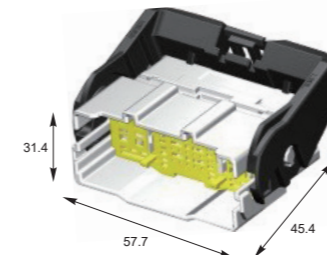
适配B型卡扣 / Mating Type B Clip
