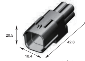
适配A型卡扣/Mating Type A Clip
