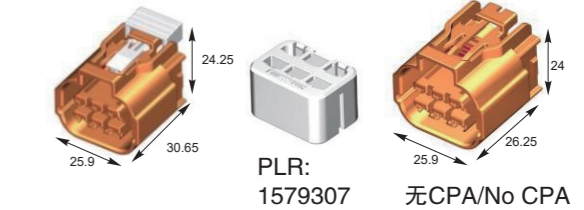
适配A型卡扣/Mating Type A Clip
